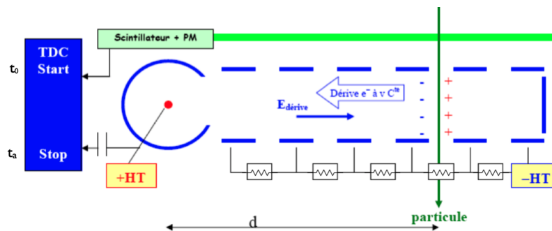
FIGURE 6.3 – Schéma illustrant le principe de fonctionnement d'une chambre à dérive.
