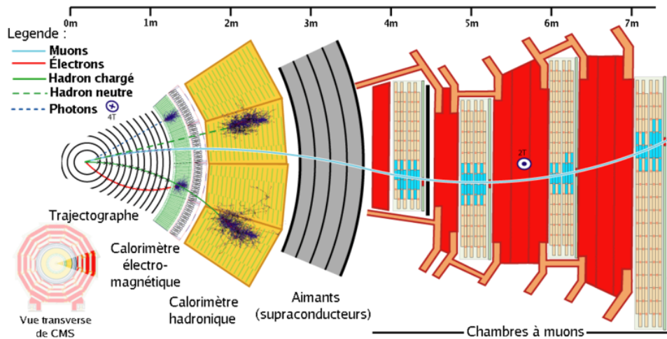
FIGURE 6.11 – Schéma général transverse du détecteur CMS. Seul 1/4 du détecteur est représenté.
