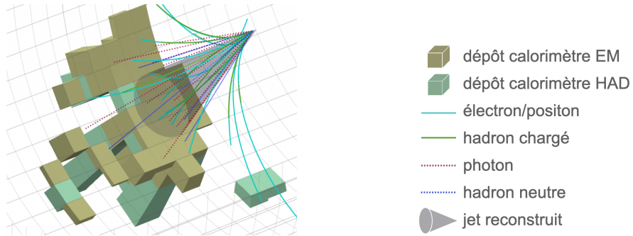
FIGURE 6.10 – Reconstruction d'un jet hadronique
