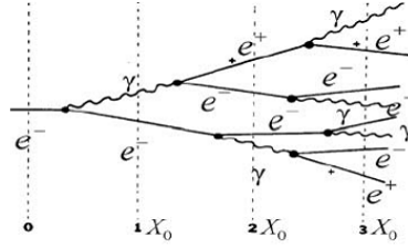
FIGURE 5.15 – Schéma d'une gerbe électromagnétique.
