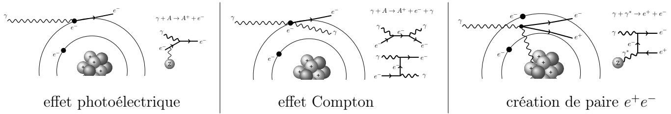
FIGURE 5.12 – Illustration des processus d'interaction d'un photon avec la matière : l'effet photoélectrique (gauche), l'effet Compton (milieu) et la création d'une paire e^+e^- (droite).
