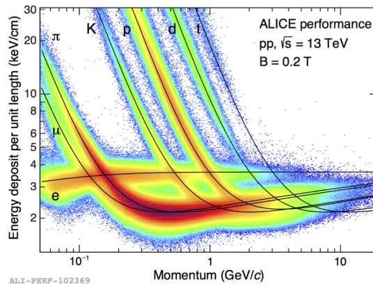
FIGURE 5.7 – Perte d'énergie par unité de longueur mesurée par l'expérience ALICE en fonction de l'impulsion. Chaque courbe noire superposée aux données correspond à l'équation de Bethe-Bloch pour une hypothèse de particule.
