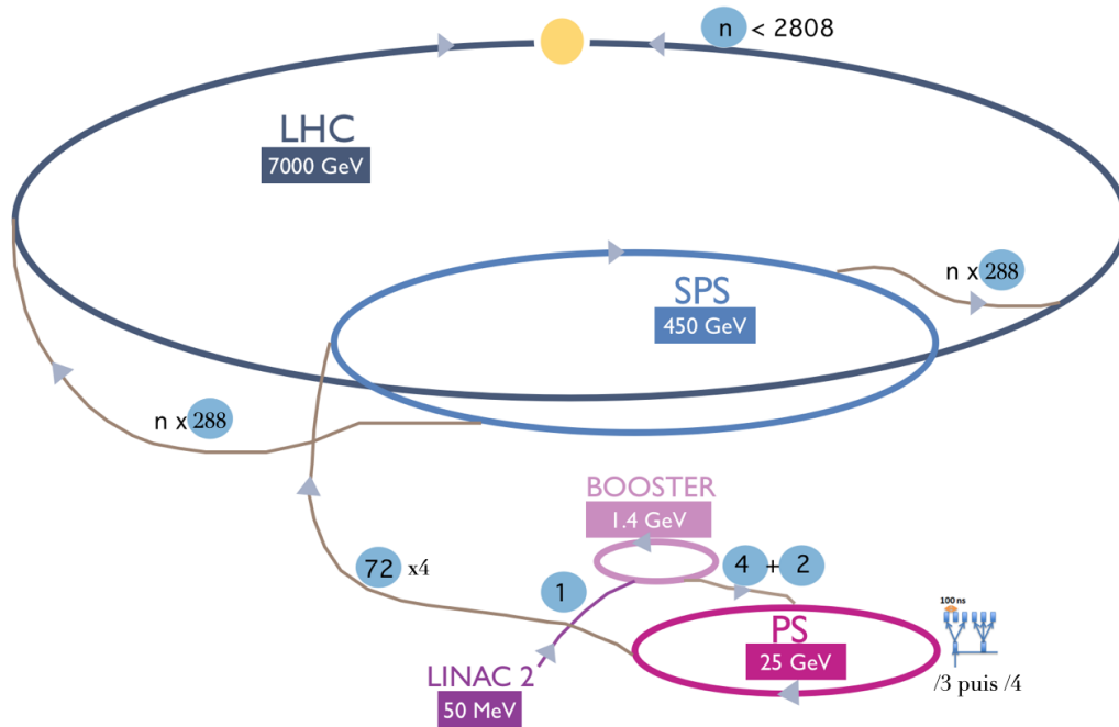
FIGURE 4.6 – Complexe d'injection des protons du LHC. Les énergies finales de chaque élément ainsi que le nombre de paquets sont indiqués.
