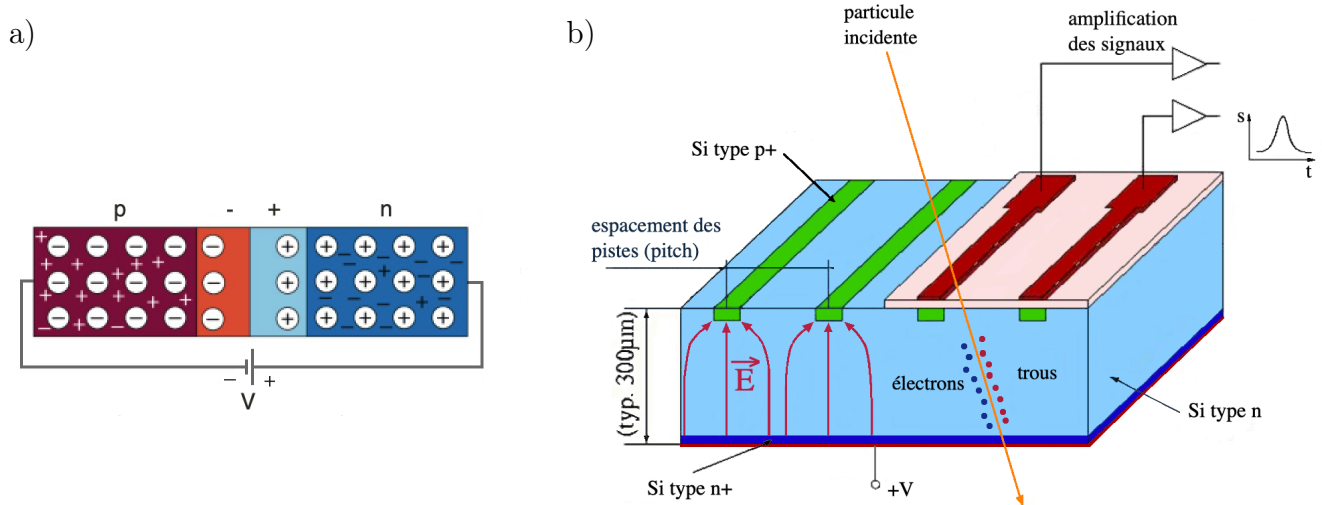
FIGURE 6.6 – A gauche : a) jonction p - n sur laquelle on applique une différence de potentiel inversée. b) schéma illustrant le principe de construction d'un détecteur à semi-conducteurs, ici au silicium (Si) avec des électrodes sous forme de pistes.
