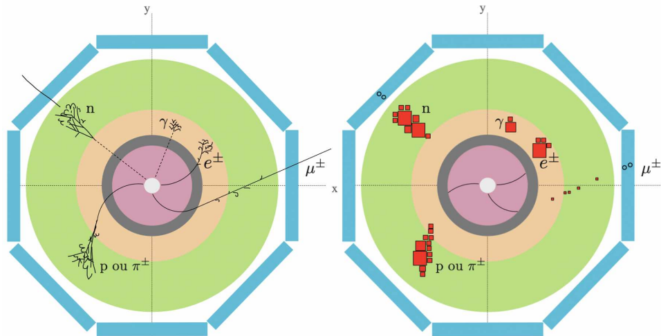
FIGURE 6.9 – a) Passage de différentes particules dans le détecteur. b) Signaux laissés par les mêmes particules : traces, dépôts d'énergie calorimétriques et impacts dans les chambres à muons. La taille des carrés est proportionnelle à l'énergie déposée localement dans les calorimètres, les cercles représentent les points d'impact dans les chambres à muons.
