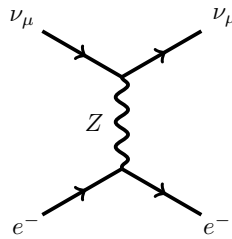
FIGURE 1.4 – Exemple de diagramme d'interaction faible à courant neutre : \nu_\mu + e^- \rightarrow \nu_\mu + e^- .
