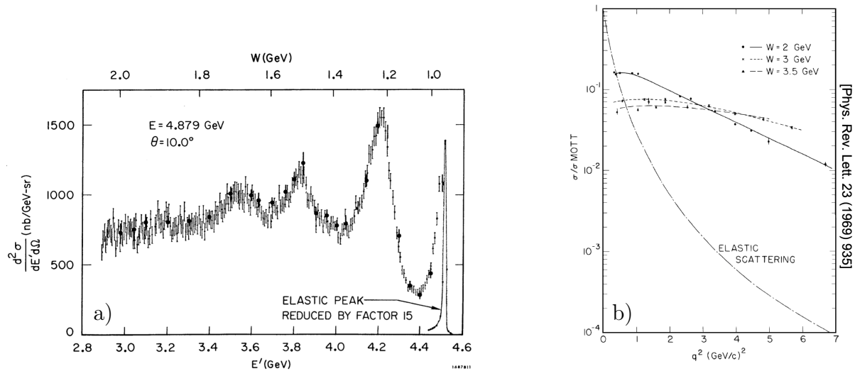
FIGURE 8.11 – a) Section efficace en fonction de la variable W (ou E' - l'énergie de l'électron diffusé), pour une angle de diffusion de 10^\circ . La pic élastique est aussi représenté mais réduit d'un facteur 15 pour la lisibilité de la figure. b) Section efficace en fonction de la variable q^2 qui dépend de l'angle de diffusion de l'électron, pour différentes valeurs de W . Les valeurs mesurées sont comparées à la courbe attendue en l'absence de centres diffuseurs de charge dans le proton (diffusion élastique).
