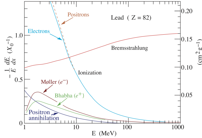
FIGURE 5.10 – Perte d'énergie moyenne par unité de longueur en fonction du produit \beta\gamma pour un électron et un positon dans du plomb.
