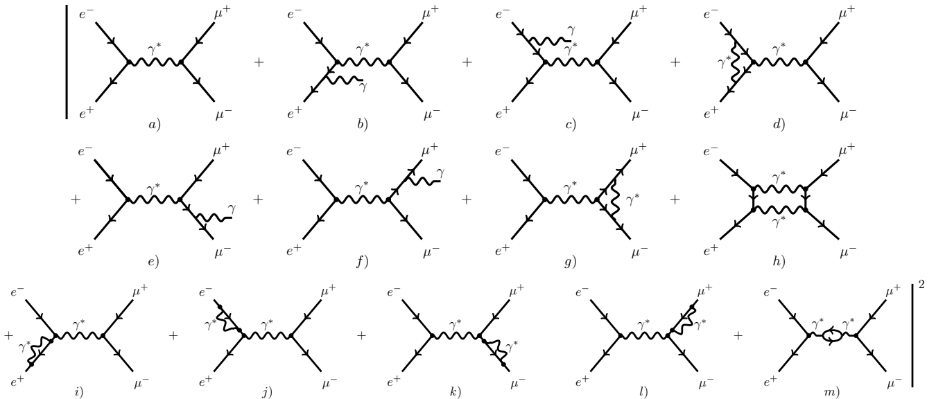
FIGURE 8.3 – Diagrammes de Feynman du processus e^+ + e^- \rightarrow \mu^+ + \mu^- à l'ordre dominant (LO) et sous dominants (NLO). La boucle du diagramme m comprend toutes paires de fermions chargés.
