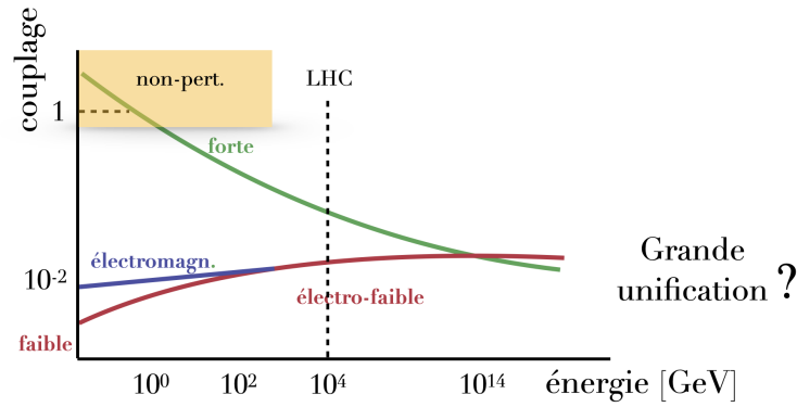
FIGURE 8.12 – Schéma illustrant les dépendances des constantes de couplage avec l'échelle d'énergie et leur extrapolation menant à la question d'une grande unification des 3 couplages.
