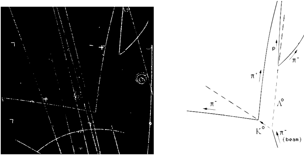
FIGURE 2.2 – gauche : cliché de chambre à bulle exposée à un faisceau de pion du Bevatron de Berkeley. droite : interprétation de l'événement : \pi^- + p \rightarrow K^0 + \Lambda^0 suivie des désintégrations K^0 \rightarrow \pi^+ + \pi^- et \Lambda^0 \rightarrow p + \pi^- .
