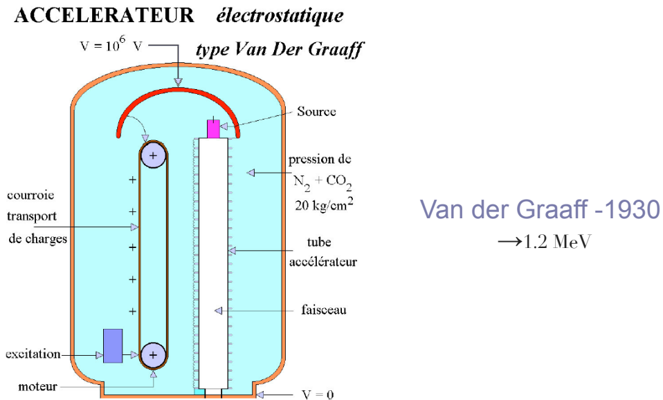
Figure 1 Schéma d'un accélérateur Van De Graaf.
