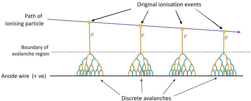
vue longitudinale
