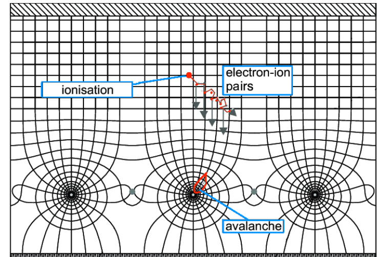
vue transverse - lignes du champ E
